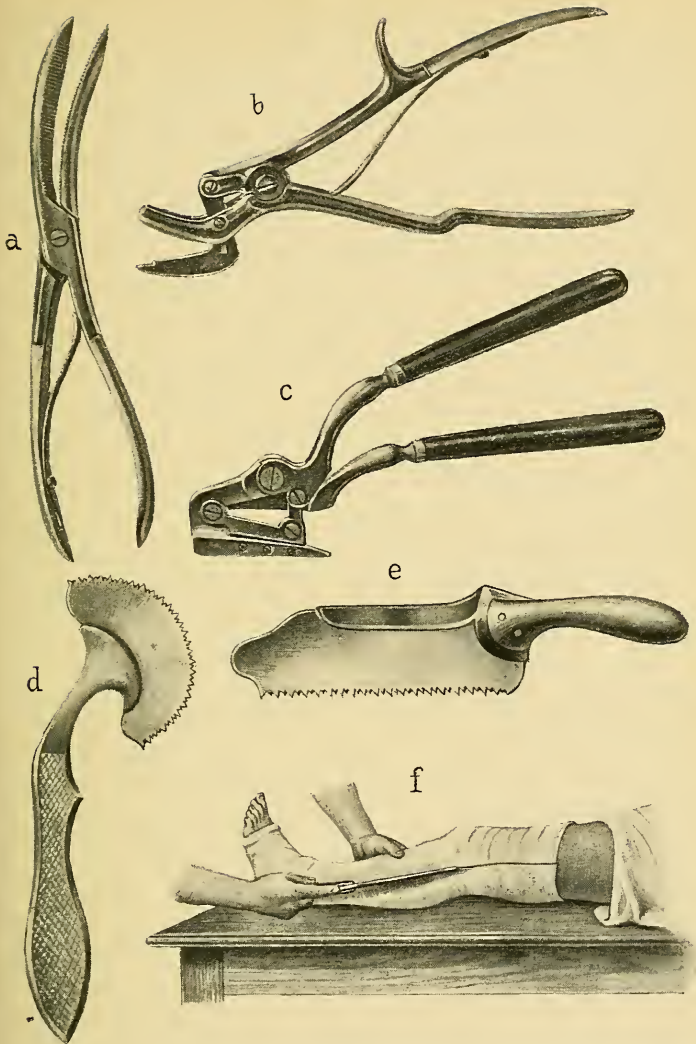
a) Zange zum Öffnen der Gypsverbände nach J. Wolff (Wolffsmaul). b) Gypsschere nach Stille. c) Gypsschere nach Empfenzeder. d) Kreis-Gypsschere. e) Blatt-Gypssäge. f) Aufsägen eines Gypsverbandes.
